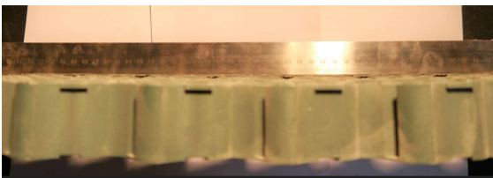
Fot. 3. Krata IP 40 po obciążeniu 57,5 kN
