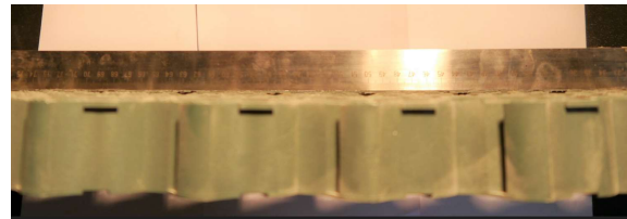
Fot. 4. Krata IP 40 po obciążeniu 80 kN
