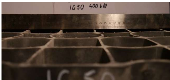
Fot. 5. Krata IG50 po obciążeniu 400 kN
