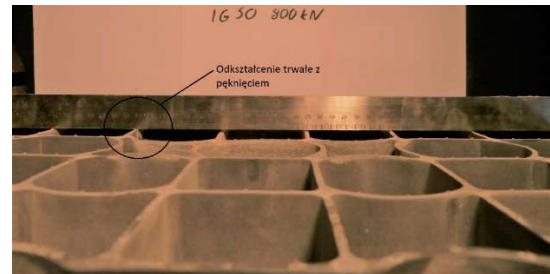
Fot. 6. Krata IG 50 po obciążeniu 800 kN
