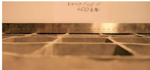
Fot. 6. Krata IG 40 Mod 1 po obciążeniu 400 kN
