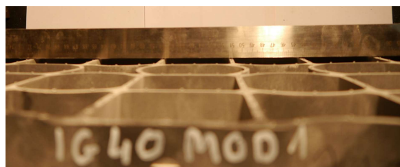
Fot. 4. Krata IG 40 Mod 1 po obciążeniu 80 kN
